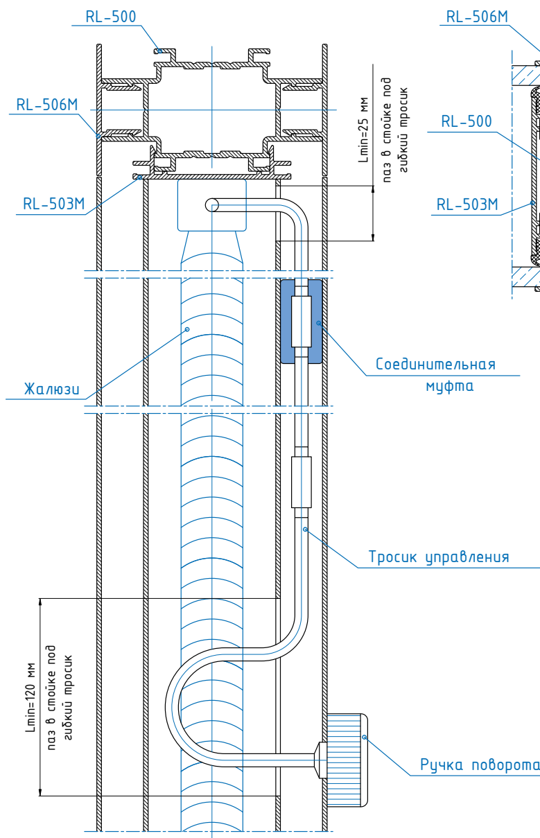
А-А
