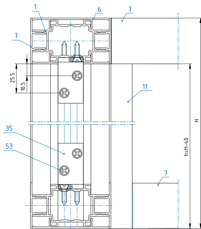
3 (RL-503M, RL-504M, заполнение условно не показаны)
