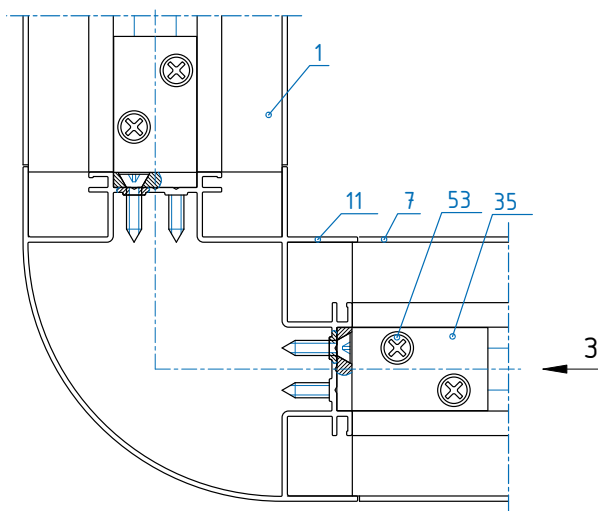
2-2 (RL-503M, RL-504M, заполнение условно не показаны)
