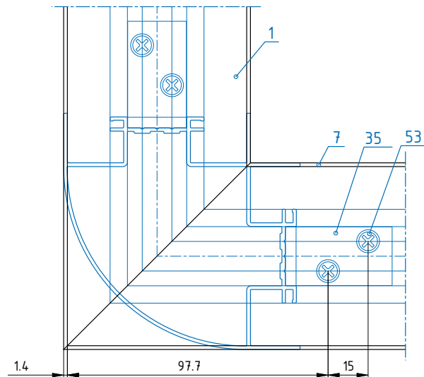
Б (RL-505M условно не показаны)
