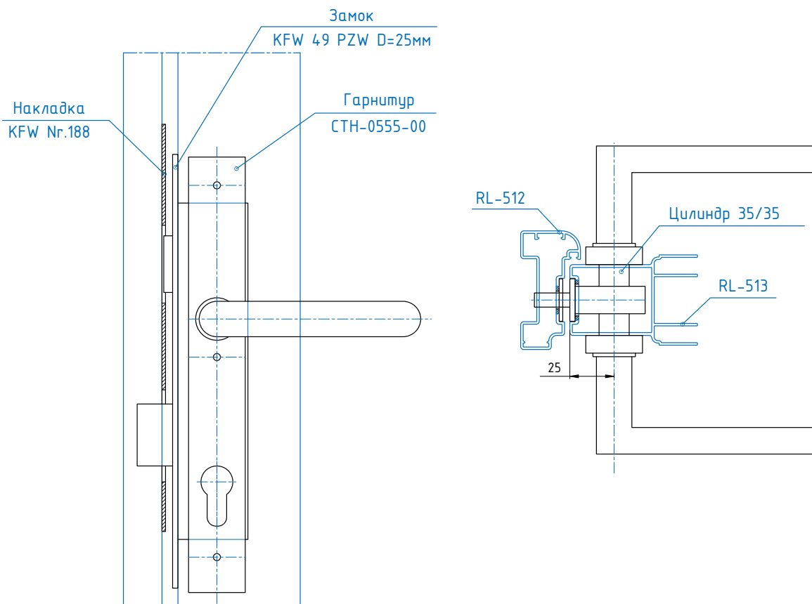
Обработка стойки RL-512
