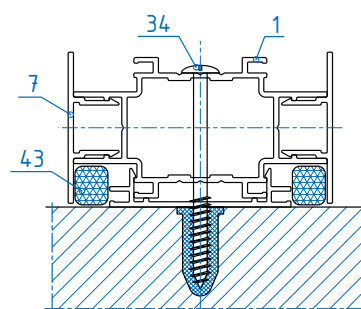
5-5 (RL-503M, RL-504M, заполнение условно не показаны)
