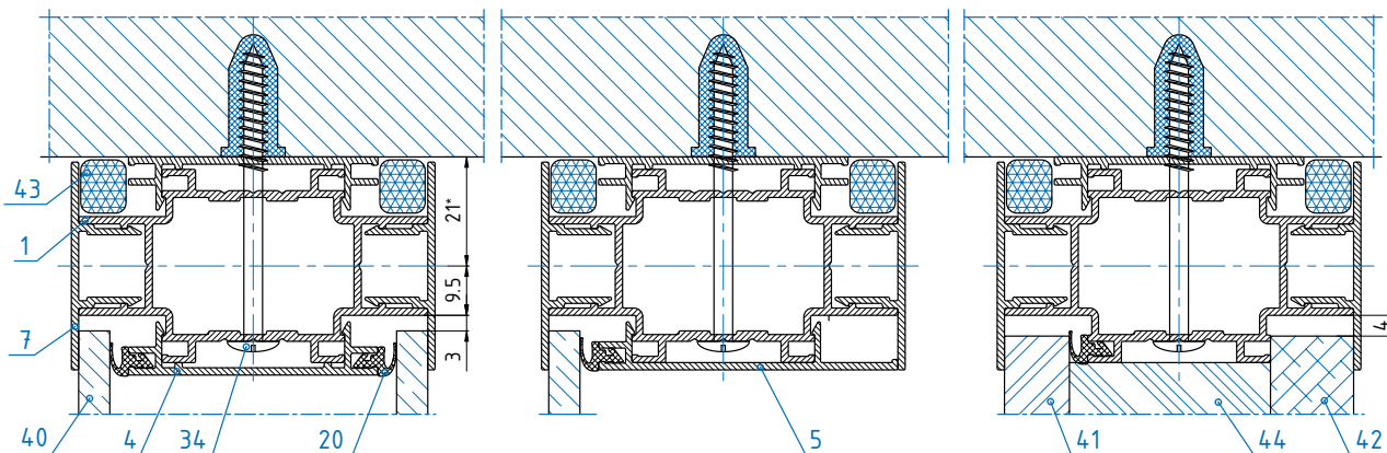
А-А
