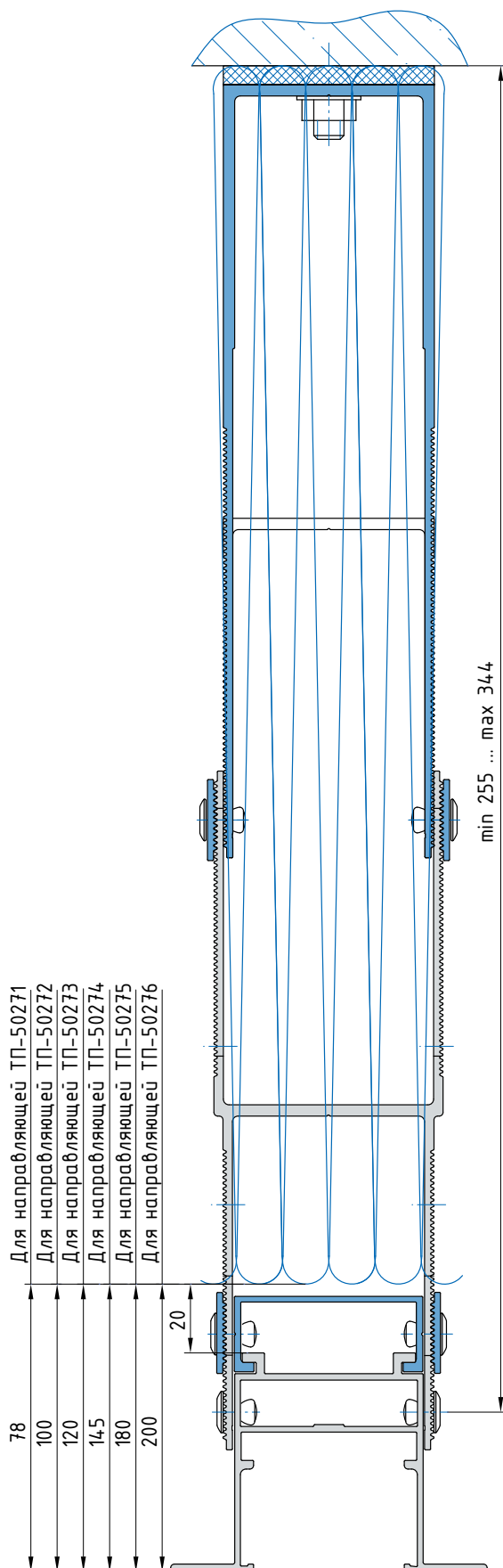
Кронштейн КП-205-...
