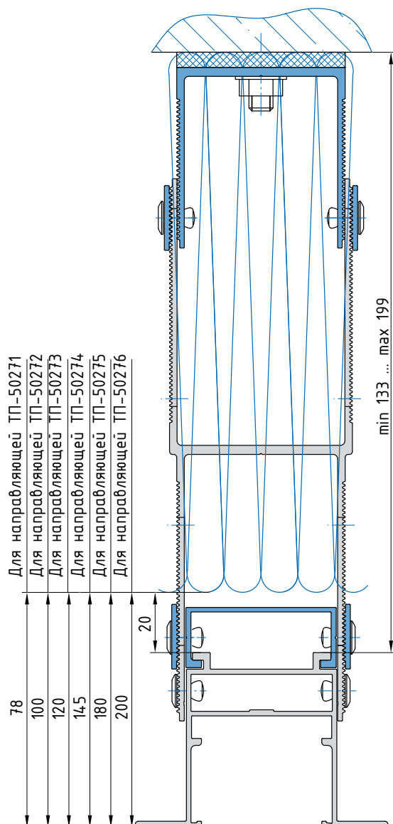
Кронштейн КП-60-...
