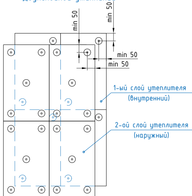
Двухслойное утепление
