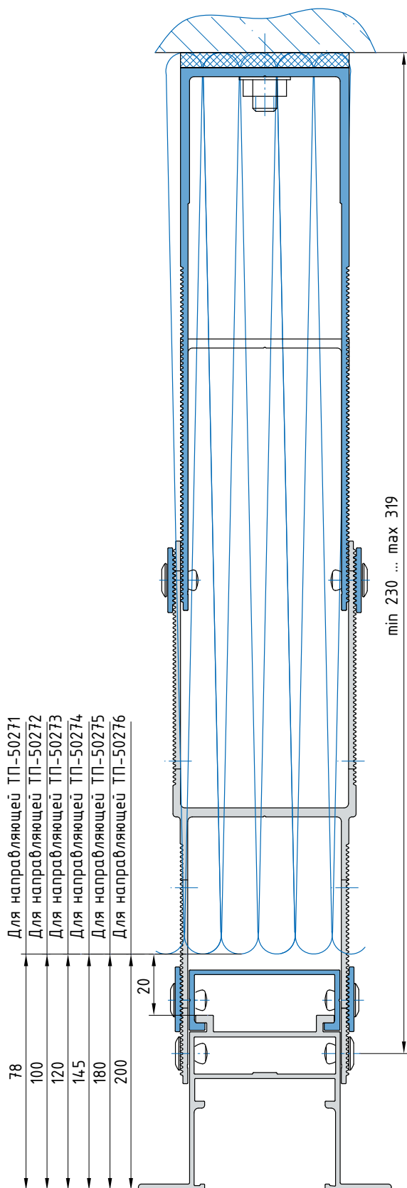
Кронштейн КП-180-...
