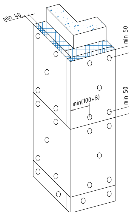
Двухслойное утепление
