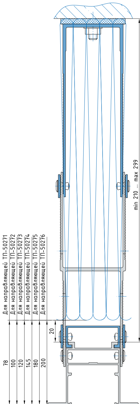
Кронштейн КП-160-...
