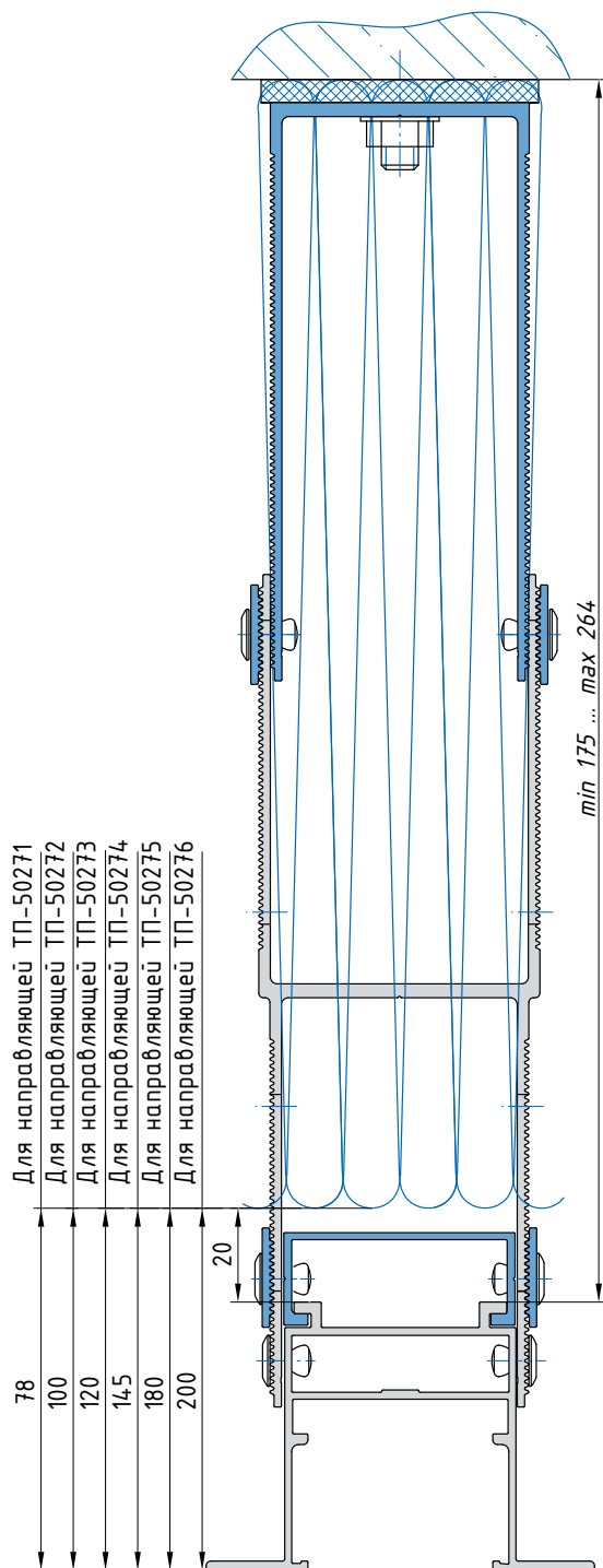
Кронштейн КП-125-...
