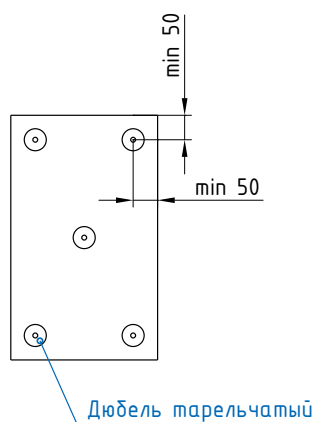
Однослойное утепление
