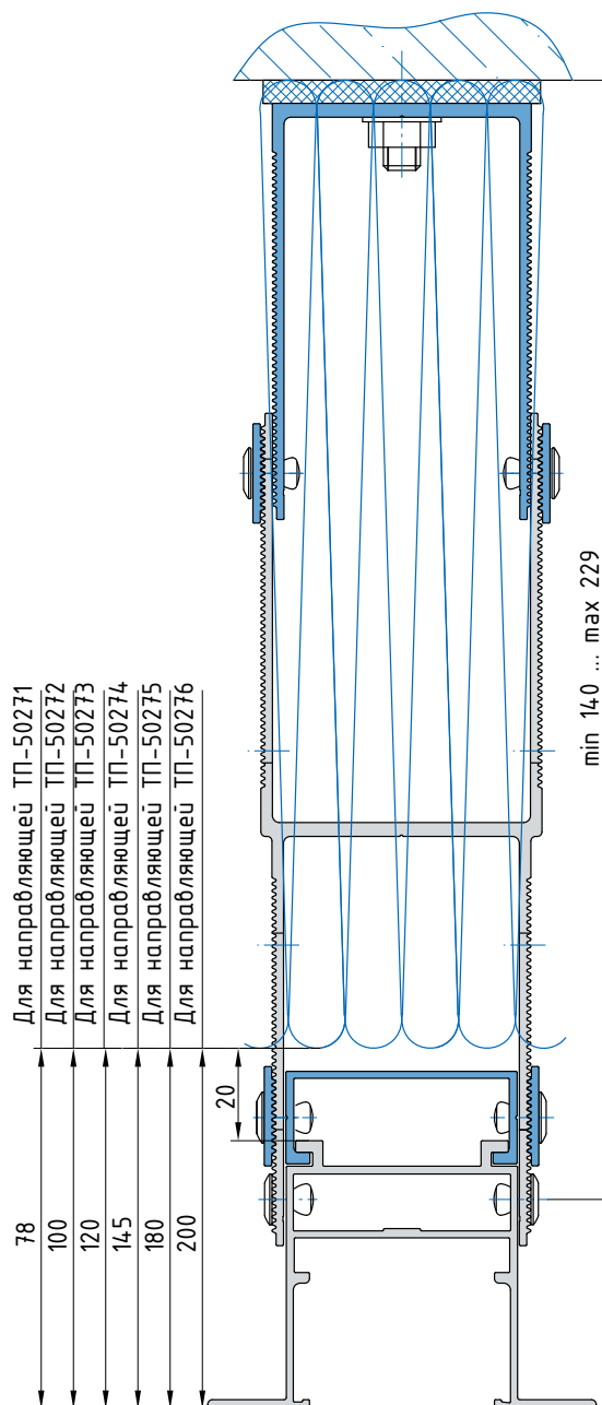
Кронштейн КП-90-...
