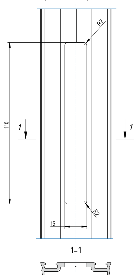
Обработка прижима
