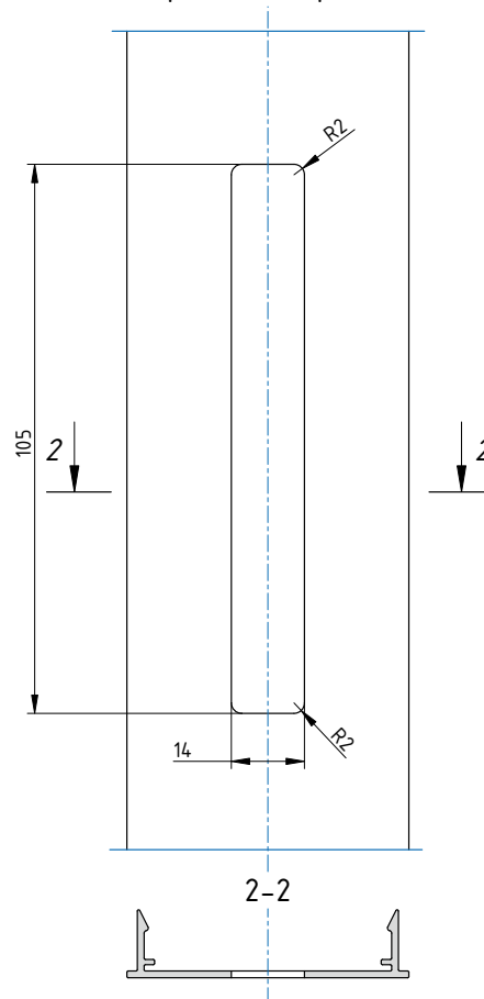
Обработка крышки
