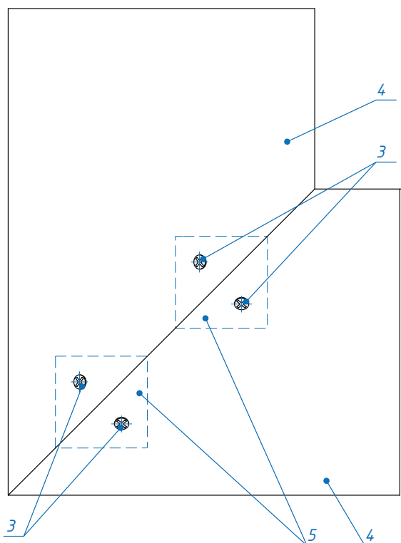
Исполнение 1
