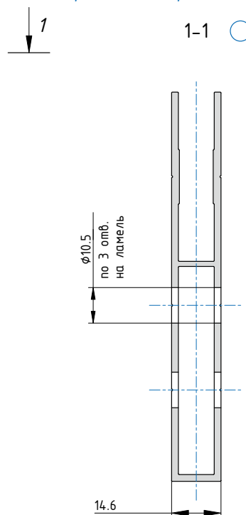
Обработка направляющей
