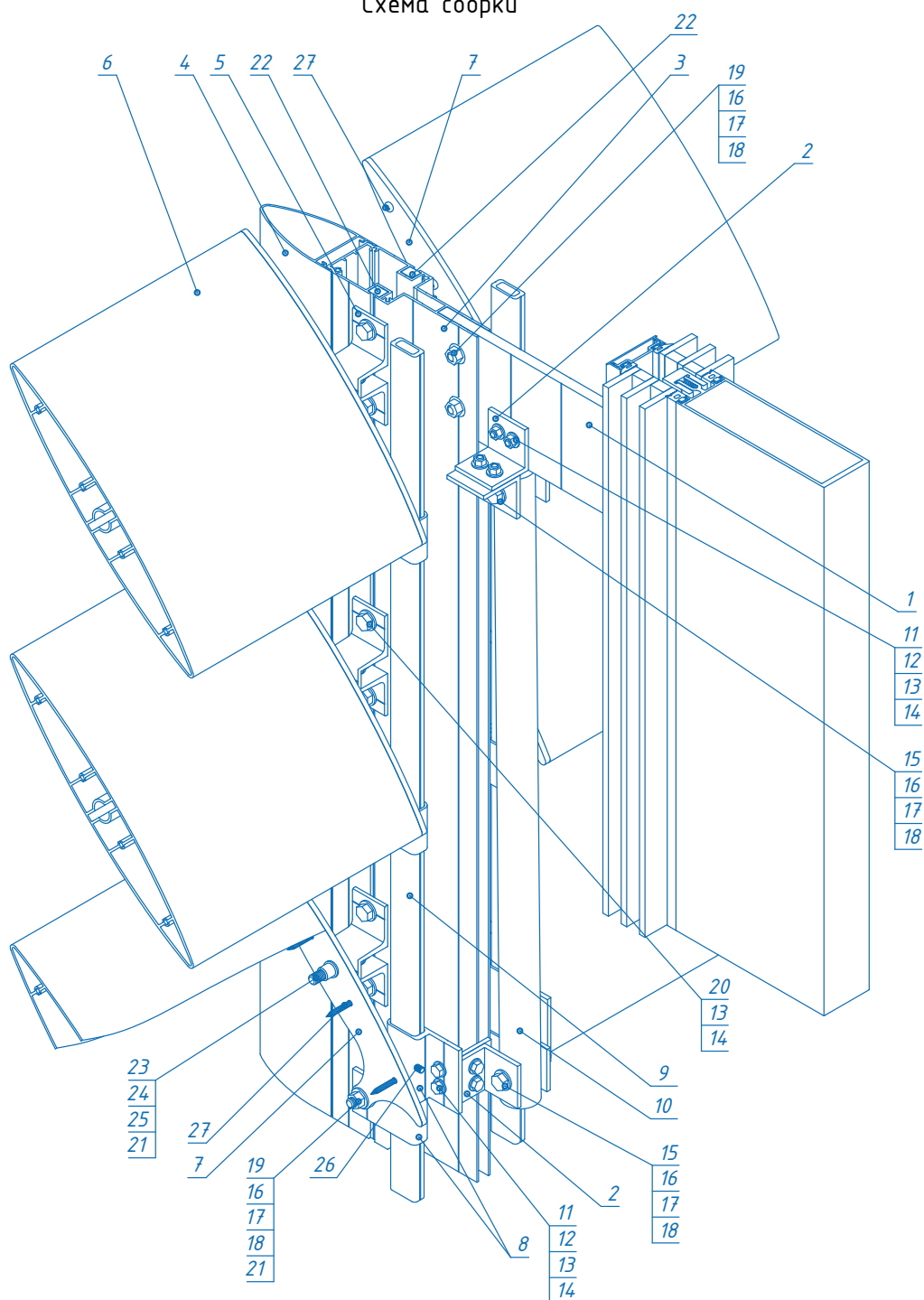
Схема сборки
