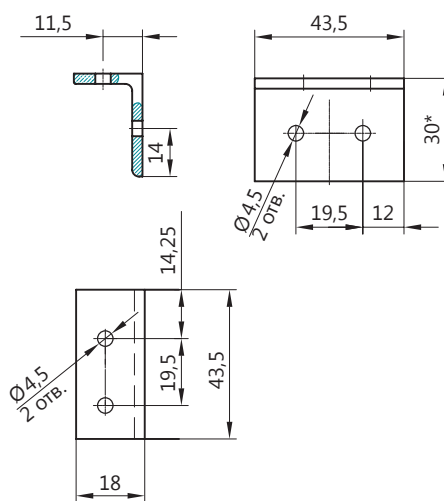
УГОЛОК 30×18×3, L=43,5 MM
