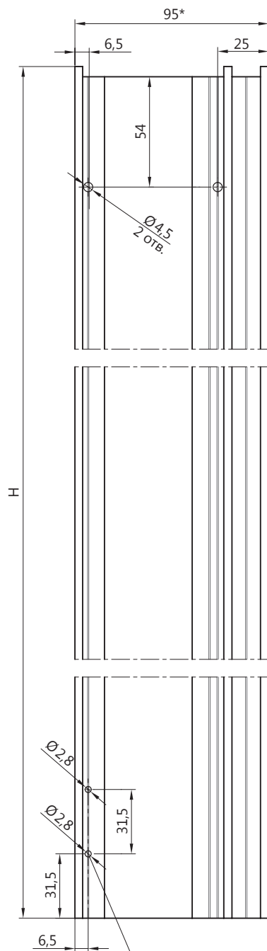
ТПТ-95.02.01
