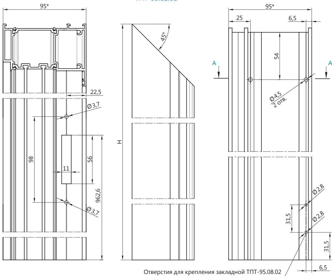
ТПТ-95.02.01
