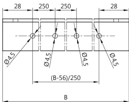
УГОЛОК 30×30×3
