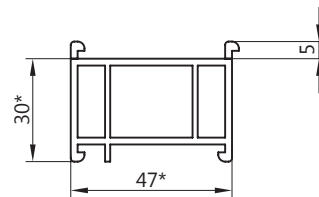
ТПУ-5769
