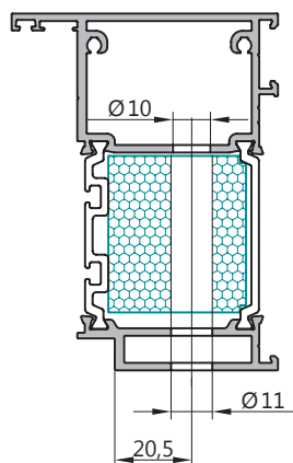
Б—Б
