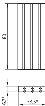
СОЕДИНИТЕЛЬ-ЗАКЛАДНАЯ ТПТ-95.08.02
