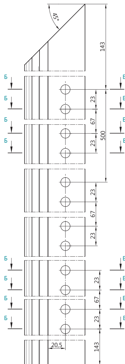
ТПТ-95.02.01
